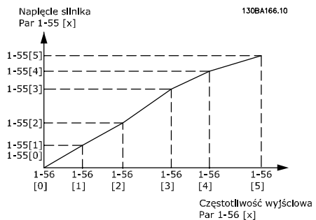
Ilustracja 4.1 Charakterystyki u/f
